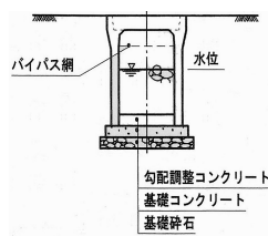
縦断図
